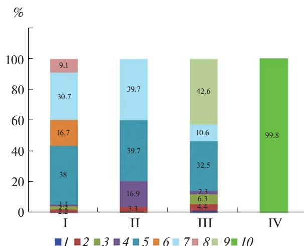
Рис. 4. Ландшафтная структура типов местности заповедника “Болонский”. I–IV– типы местности (см. легенду рис. 3); 1–10 – доминирующие растительные сообщества: Урочищ низких релок и береговых валов: 1 – широколиственно-мелколиственные леса; 2 – мелколиственные леса в сочетании с ерниковыми зарослями, травяными лугами и низинными болотами; 3 – мелколиственно-лиственничное редколесье в сочетании с ерниковыми зарослями, влажными и сырыми травяными лугами и низинными болотами; 4 – ерниковые заросли в сочетании с угнетенным белоберезово-лиственнично-ольховым редколесьем. Урочищ окраин релок и прилегающих слабонаклонных поверхностей: 5 – кустарниково-вейниково-осоковые заболоченные луга в сочетании с травяными, травяно-моховыми и моховыми болотами. Урочищ плоских горизонтальных поверхностей: 6 – травяные луга и болота; 7 – мохово-травяные болота; 8 – закустаренные травяные луга и болота; 9 – кустарничково-травяно-моховые грядово-мочажинные (с разной долей участия гряд и мочажин) и грядово-ложбинные болота. Урочищ поймы: 10 – ивняково-травяные комплексы низкой сырой и заболоченной поймы.
